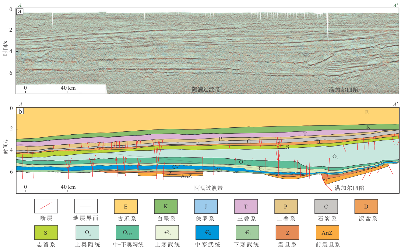
图4 塔里木盆地阿满过渡带区域地质剖面(剖面位置见图1)
