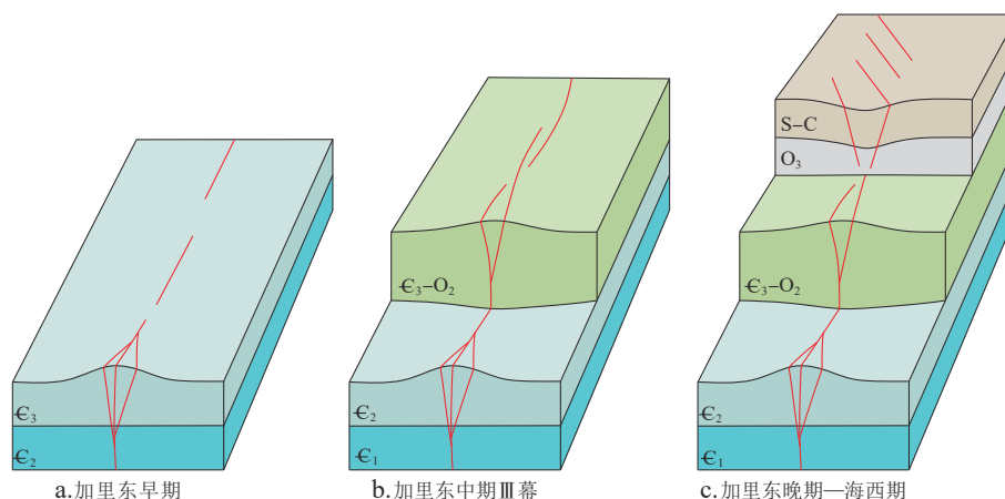
图 12 富满油田东部走滑断裂演化模式
