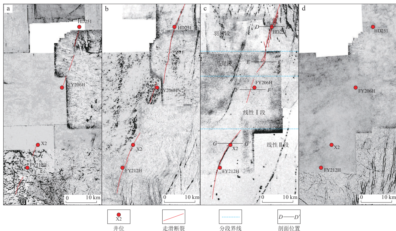
图8 富满油田F 12 走滑断裂三维多层相干切片
