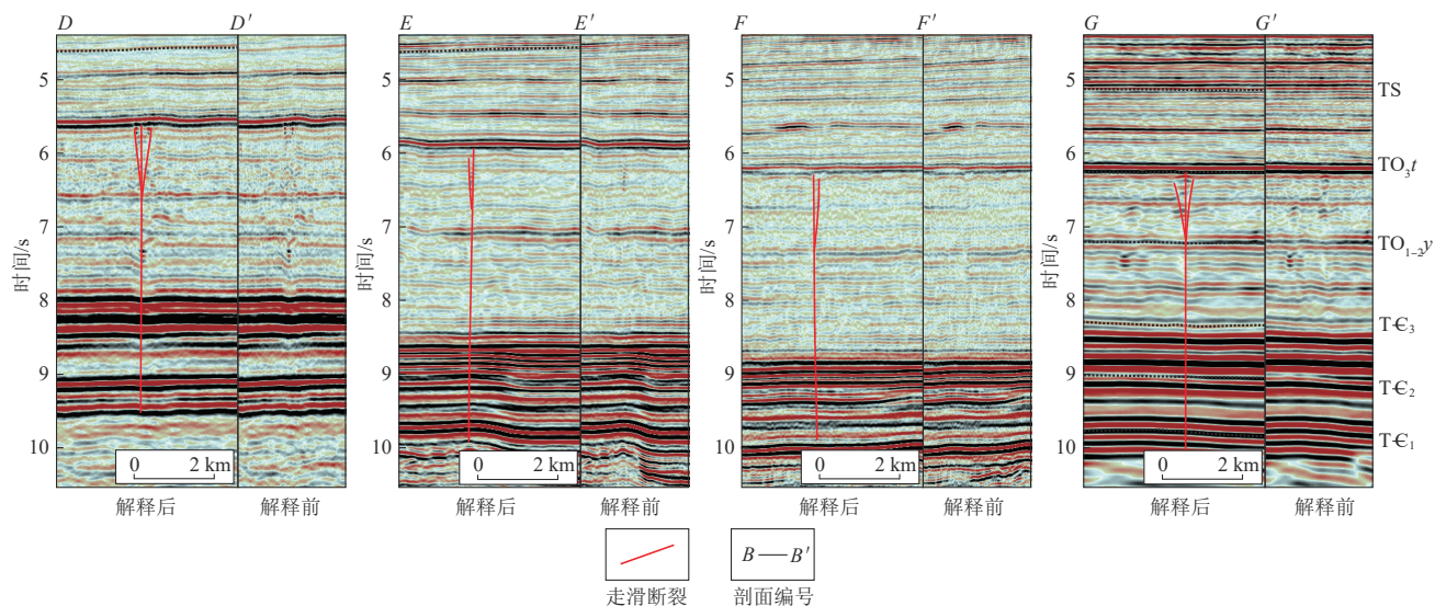
图9 富满油田F 12 走滑断裂分段变形特征(剖面位置见图8)
